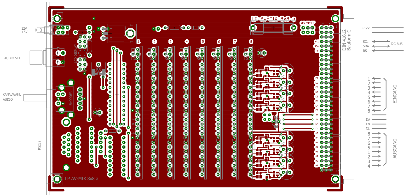
Leiterplatte LP AV-MIX-8x8 a
