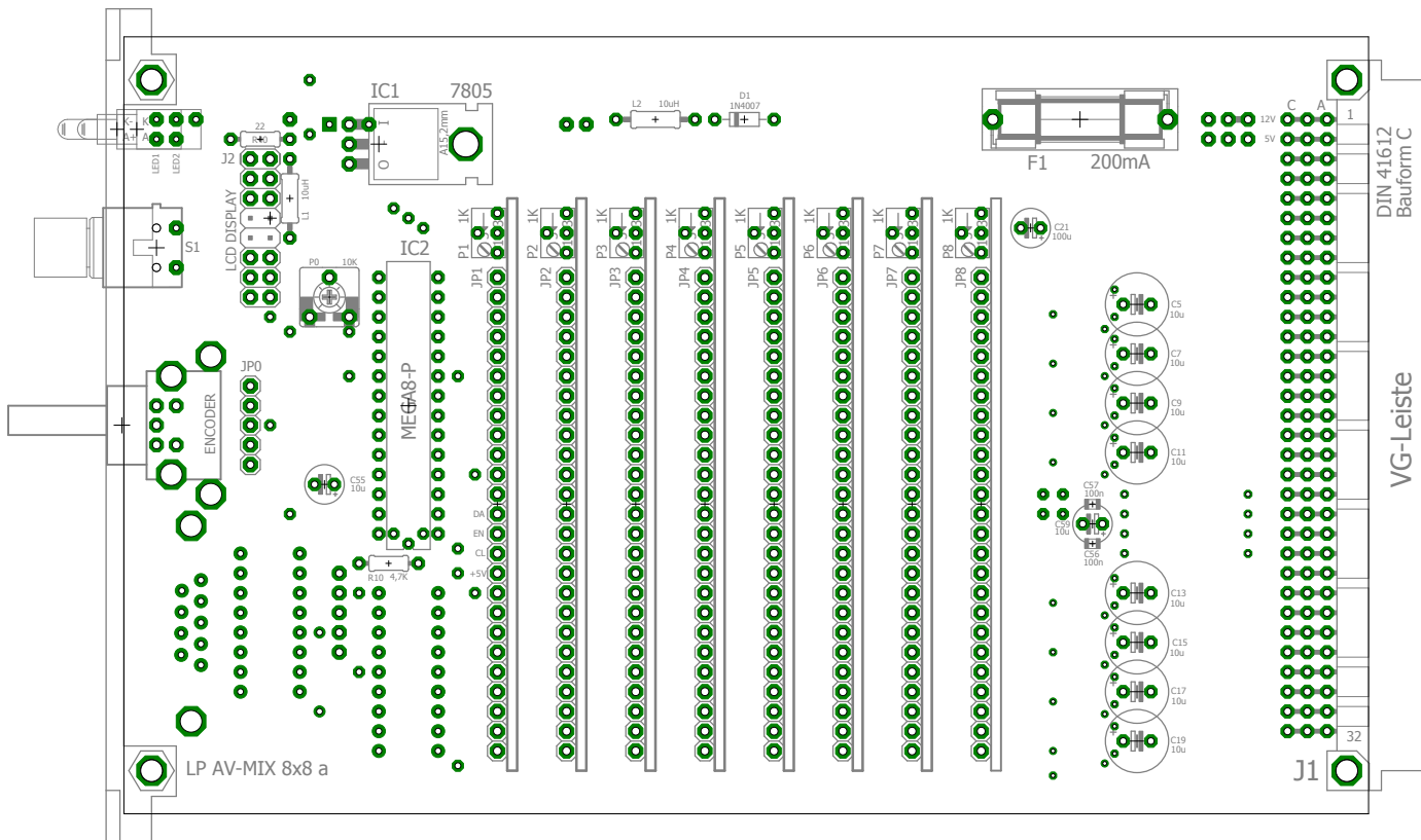
Leiterplatte LP AV-MIX-8x8 a
