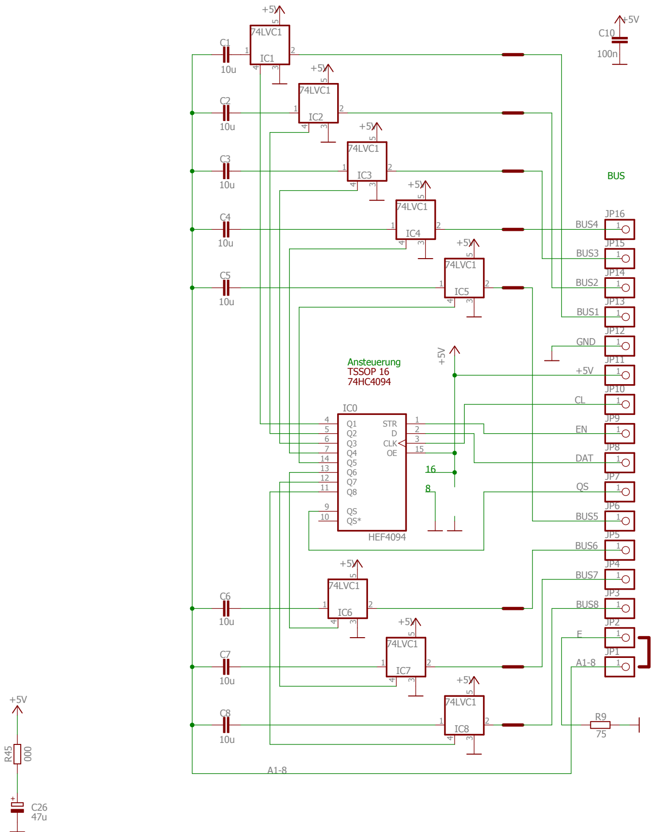
Leiterplatte LP-AVMIX-SCH
