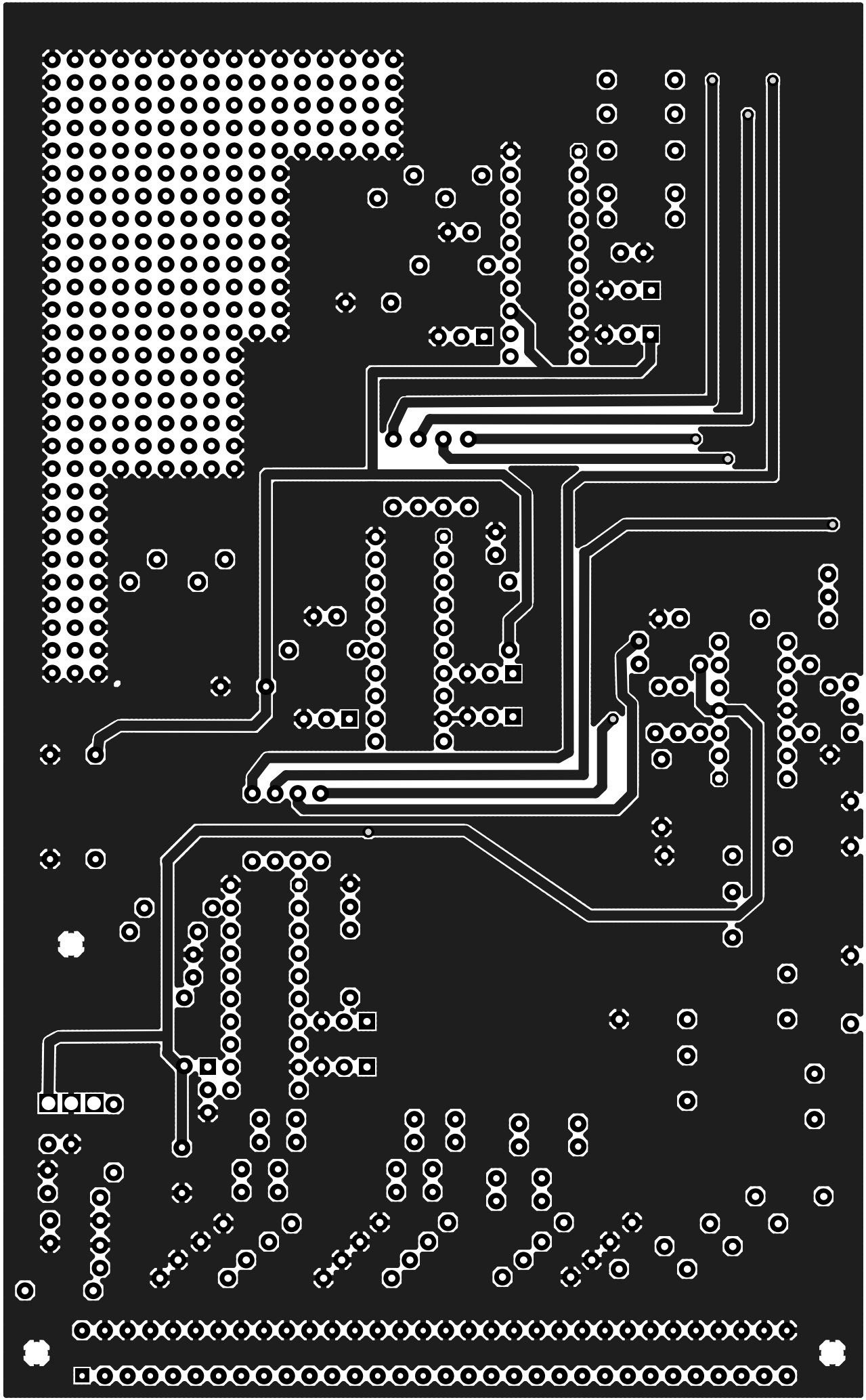
Platinenoberseite
